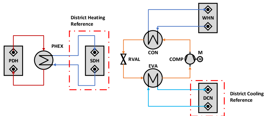
Abbildung 37: Schema des Referenzsystems, bestehend aus Fernwärmeübergabestation und Kompressionskältemaschine
