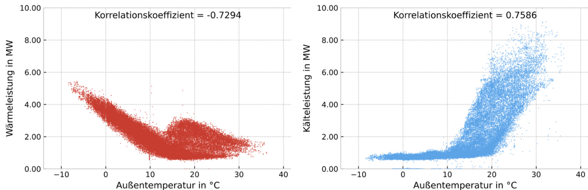
Abbildung 24: Korrelationsanalyse für Wärme und Kälte in Abhängigkeit der Außentemperatur nach Bittner [62]
