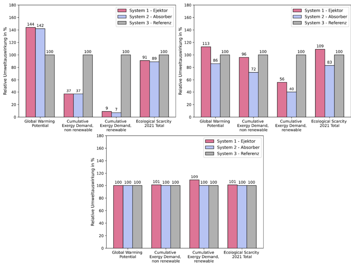
Überblick über die Umweltauswirkungen der einzelnen Varianten: Nur-Kühlen (Sommer, Fall a (oben links)), Heizen und Kühlen (Übergangszeit, Fall b (oben rechts)) und Nur-Heizen (Winter, Fall c (unten mittig))
