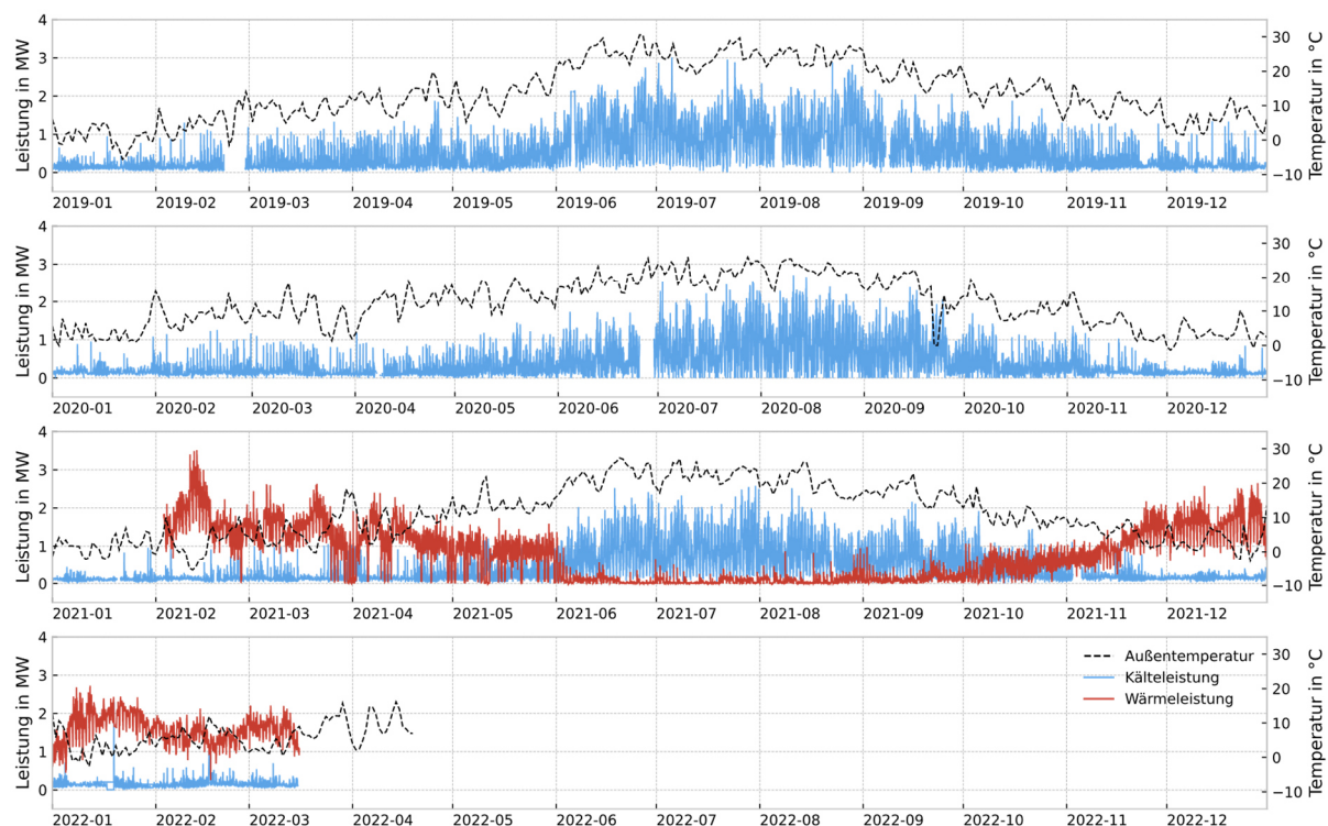
Abbildung 15: Lastgänge und Außentemperaturverläufe des Bürokomplexes für 2019 bis 2022 nach Bittner [62]
