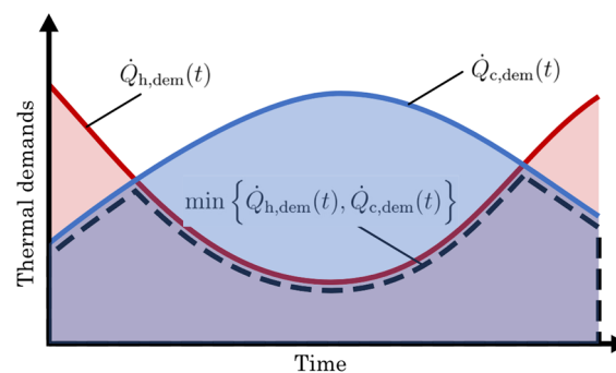
Abbildung 14: Wärme- ( \dot{Q}_{h,dem}(t) in rot) und Kältebedarf ( \dot{Q}_{c,dem}(t) in blau) sind über die Zeit dargestellt. Der Demand Overlap Coefficient (DOC) quantifiziert die Überschneidung beider Bedarfe zum Zeitpunkt t durch \min\{\dot{Q}_{h,dem}(t), \dot{Q}_{c,dem}(t)\} (schwarz strichlierte Linie) nach Wirtz et al. [68]
