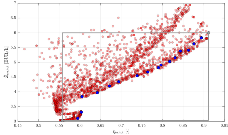
Abbildung 41: Pareto-Front der zweiten Absorberschaltungsvariante für die simultane Wärme- und Kältebereitstellung
