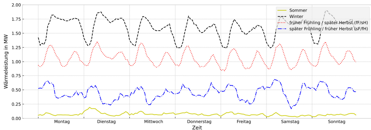
Abbildung 19: Typischer Wochen-Lastgang des Bürokomplexes für Wärme nach Bittner [62]
