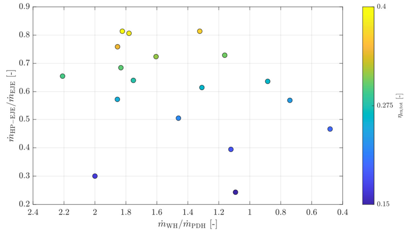
Abbildung 48: Parameterraum der zweiten Ejektorschaltungsvariante für die simultane Wärme- und Kältebereitstellung
