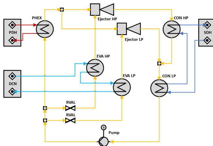
Abbildung 34: Schema des Ejektorkreislaufs zur reinen Kältebereitstellung
