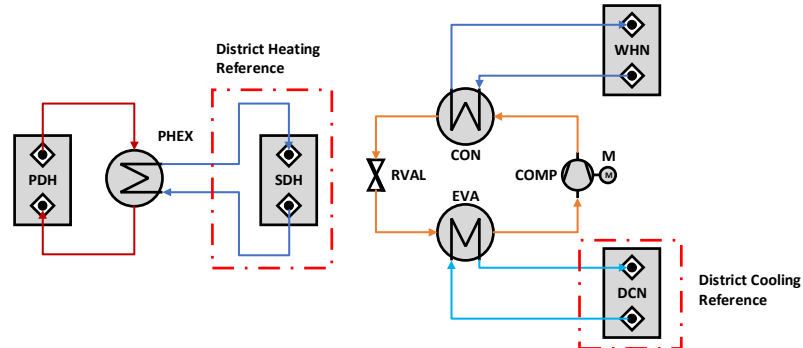
Abbildung 52: Schema des Referenzsystems im Falle der simultanen Wärme- und Kältebereitstellung
