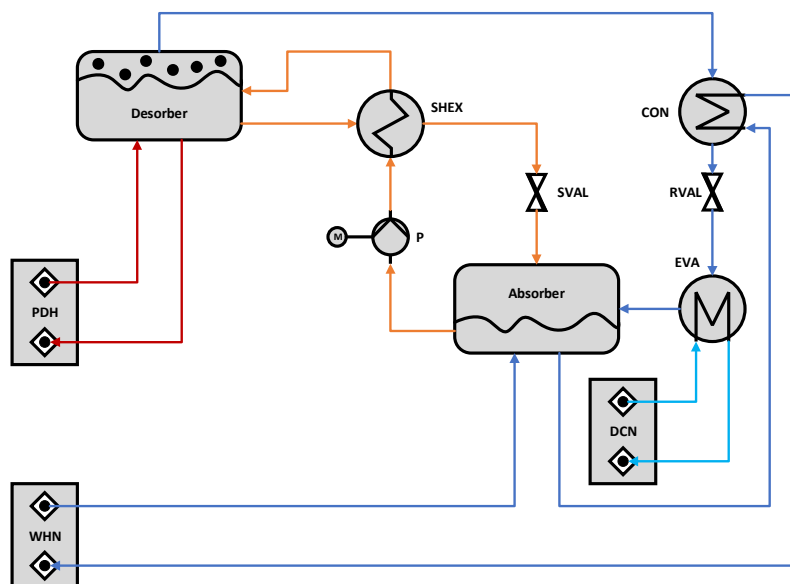
Abbildung 31: Schema des Absorptionswärmetauscher zur reinen Kältebereitstellung
