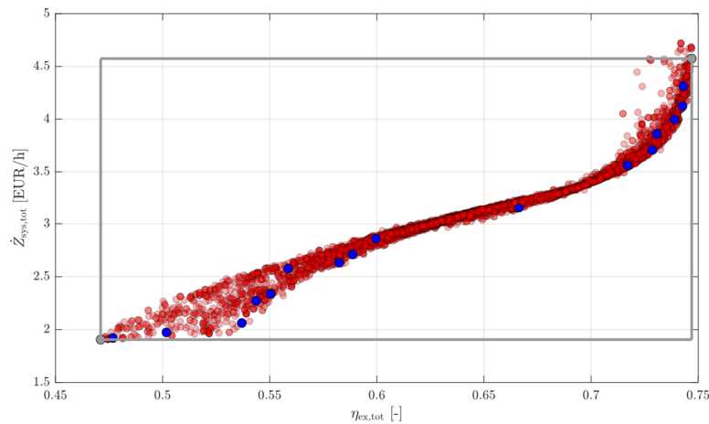
Abbildung 43: Pareto-Front der dritten Absorberschaltungsvariante für die reine Wärmebereitstellung
