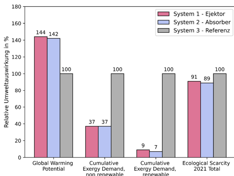
Abbildung 54: Relative Umweltauswirkungen der drei Systeme im Vergleich, Variante 1 - Reine Kältebereitstellung
