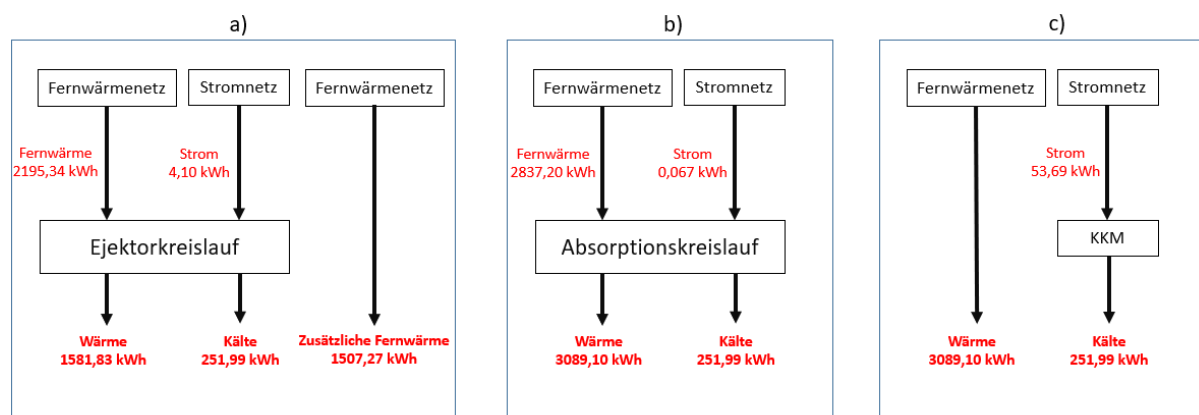
Abbildung 38: Variante 2: stündliche Energieinputs und - outputs. für den Vergleich der 3 Systeme mit Systemerweiterungsansatz. a) System 1 – Ejektorschaltung; b) System 2 - Absorberschaltung; c) System 3 – Referenzsystem.
