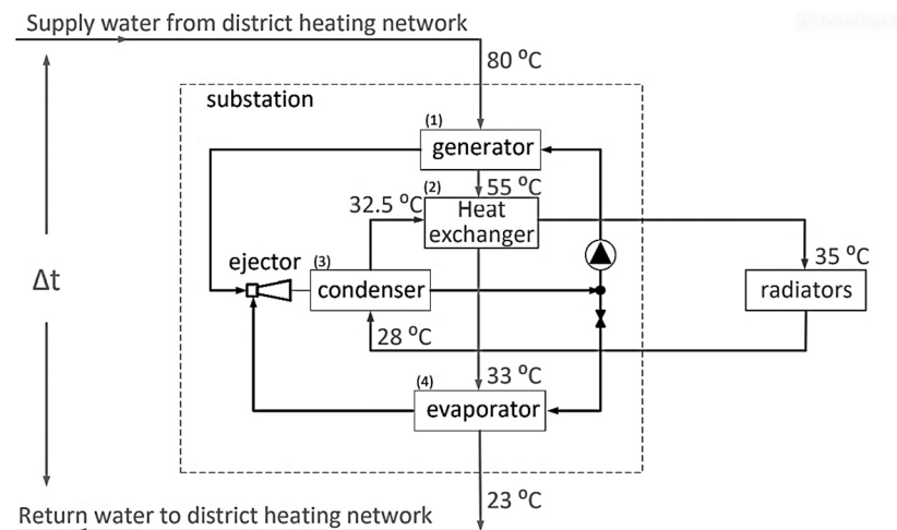
Abbildung 10: Schema eines Ejektorprozesses zur Absenkung der primären Rücklauftemperatur in einem Fernwärmenetz nach Fang [47]
