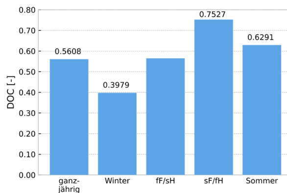
Abbildung 26: Demand Overlap Coefficient für das Krankenhaus nach Bittner [62]
