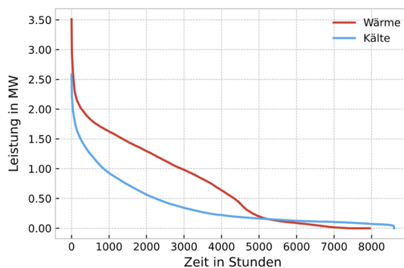
Abbildung 17: Jahresdauerlinie für Wärme und Kälte im Jahr 2021 nach Bittner [62]
