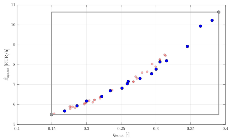
Abbildung 47: Pareto-Front der zweiten Ejektorschaltungsvariante für die simultane Wärme- und Kältebereitstellung
