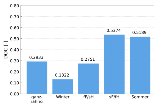
Abbildung 18: Demand Overlap Coefficient für den Bürokomplex nach Bittner [62]
