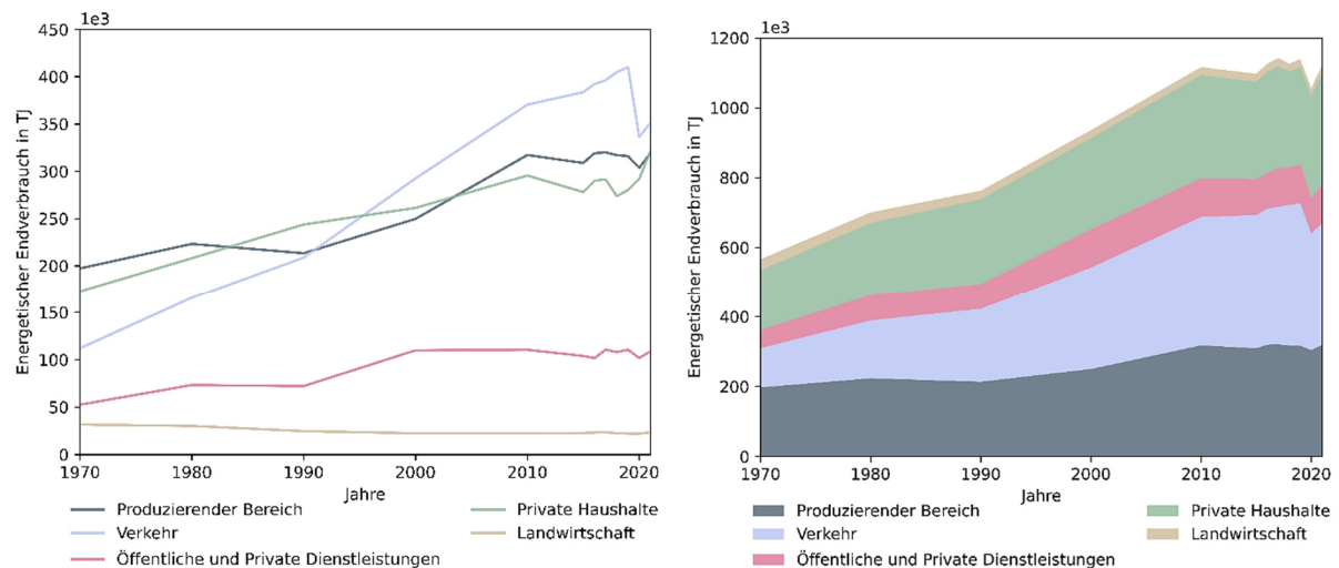
Abbildung 3: Energetischer Endverbrauch in Österreich nach Sektoren von 1970 bis 2021 (Links: einzelne Verläufe der Sektoren; Rechts: gestapelter Verlauf der Sektoren nach Statistik Austria [10])
