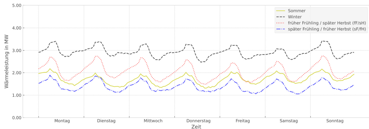
Abbildung 27: Typischer Wochen-Lastgang des Krankenhauses für Wärme nach Bittner [62]
