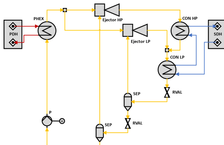
Abbildung 36: Schema des Ejektorkreislaufs zur reinen Wärmebereitstellung
