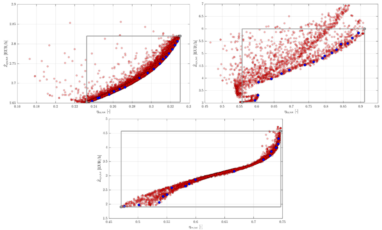
Pareto-Fronten der ersten Absorberschaltungsvariante (oben links), der zweiten Absorberschaltungsvariante (oben rechts) und der dritten Absorberschaltungsvariante (unten mittig)
