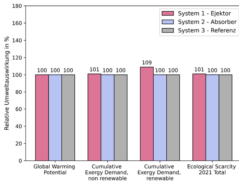
Abbildung 56: Relative Umweltauswirkungen der drei Systeme im Vergleich, Variante 3 - Reine Wärmebereitstellung
