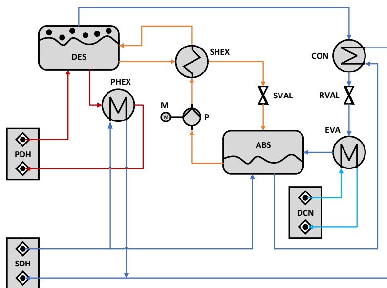
Abbildung 32: Schema des Absorptionswärmetauschers zur simultanen Wärme- und Kältebereitstellung
