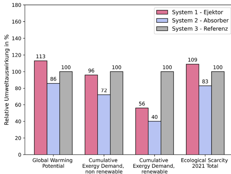
Abbildung 55: Relative Umweltauswirkungen der drei Systeme im Vergleich, Variante 2 – Simultane Wärme- und Kältebereitstellung
