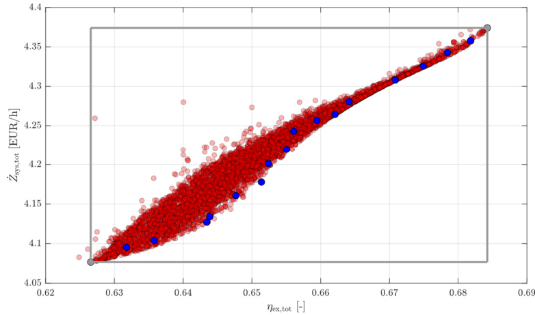
Abbildung 49: Pareto-Front der dritten Ejektorschaltungsvariante für die reine Wärmebereitstellung
