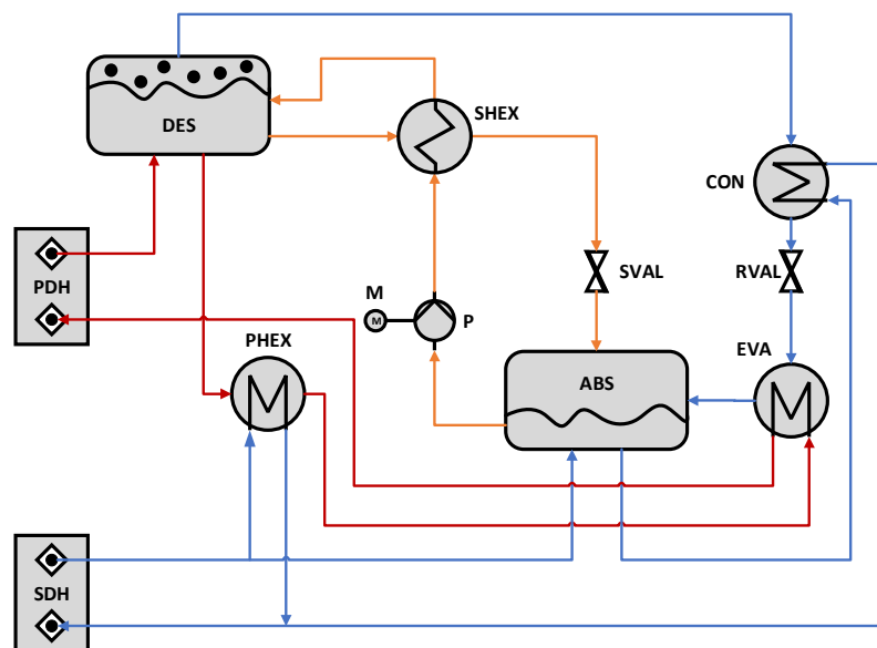
Abbildung 33: Schema des Absorptionswärmetauschers zur reinen Wärmebereitstellung
