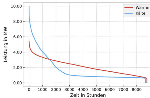
Abbildung 25: Jahresdauerlinie für Wärme und Kälte im Jahr 2021 nach Bittner [62]
