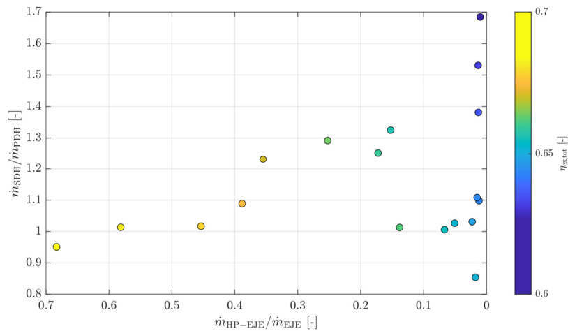
Abbildung 50: Parameterraum der dritten Ejektorschaltungsvariante für die reine Wärmebereitstellung
