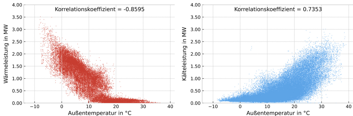
Abbildung 16: Korrelationsanalyse für Wärme und Kälte in Abhängigkeit der Außentemperatur nach Bittner [62]
