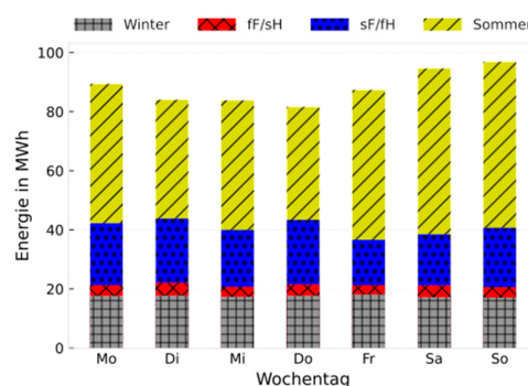
Abbildung 30: Typische tägliche Kälteenergiemenge des Krankenhauses nach Bittner [62]
