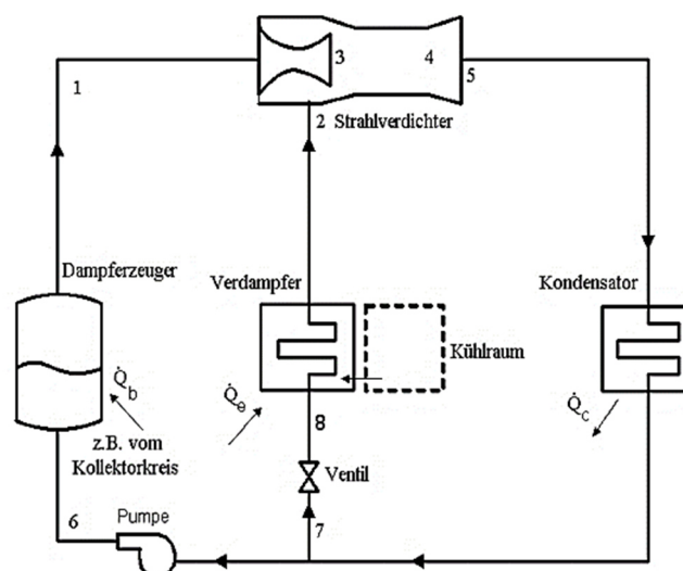
Abbildung 11: Schema einer Dampfstrahlkälteanlage mit einem Dampferzeuger nach Izuba [49]
