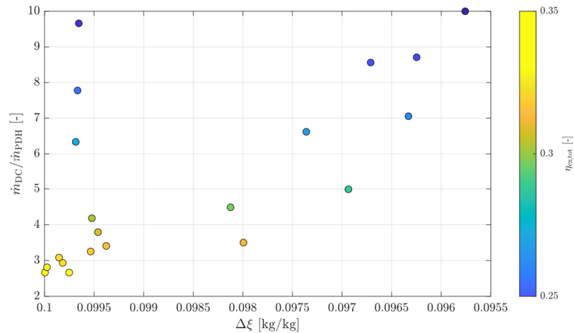
Abbildung 40: Parameterraum der ersten Absorberschaltungsvariante für die reine Kältebereitstellung
