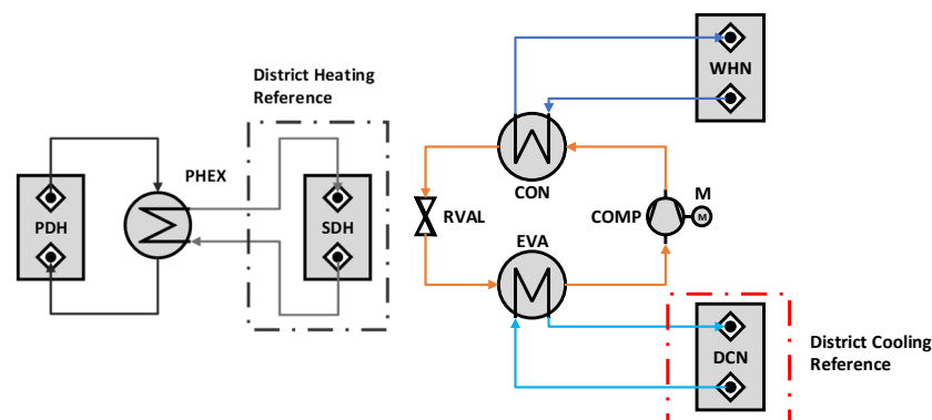
Abbildung 51: Schema des Referenzsystems im Falle der reinen Kältebereitstellung
