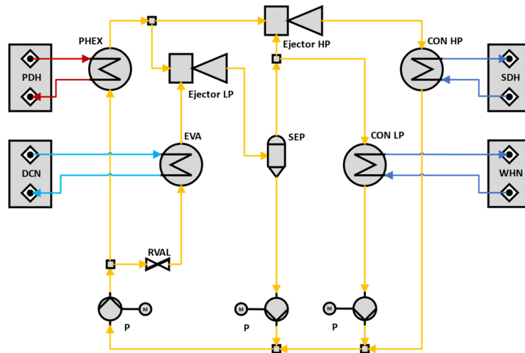
Abbildung 35: Schema des Ejektorkreislaufs zur simultanen Wärme- und Kältebereitstellung
