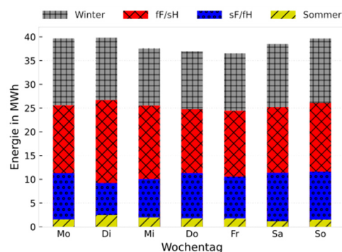
Abbildung 20: Typische tägliche Wärmeenergiemengen des Bürokomplexes nach Bittner [62]
