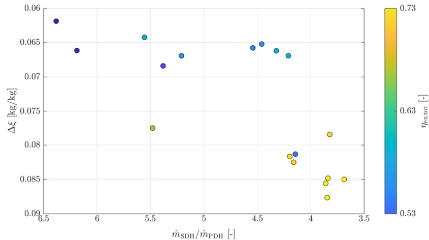
Abbildung 44: Parameterraum der dritten Absorberschaltungsvariante für die reine Wärmebereitstellung
