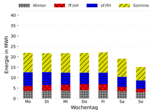
Abbildung 22: Typische tägliche Kälteenergiemengen des Bürokomplexes nach Bittner [62]
