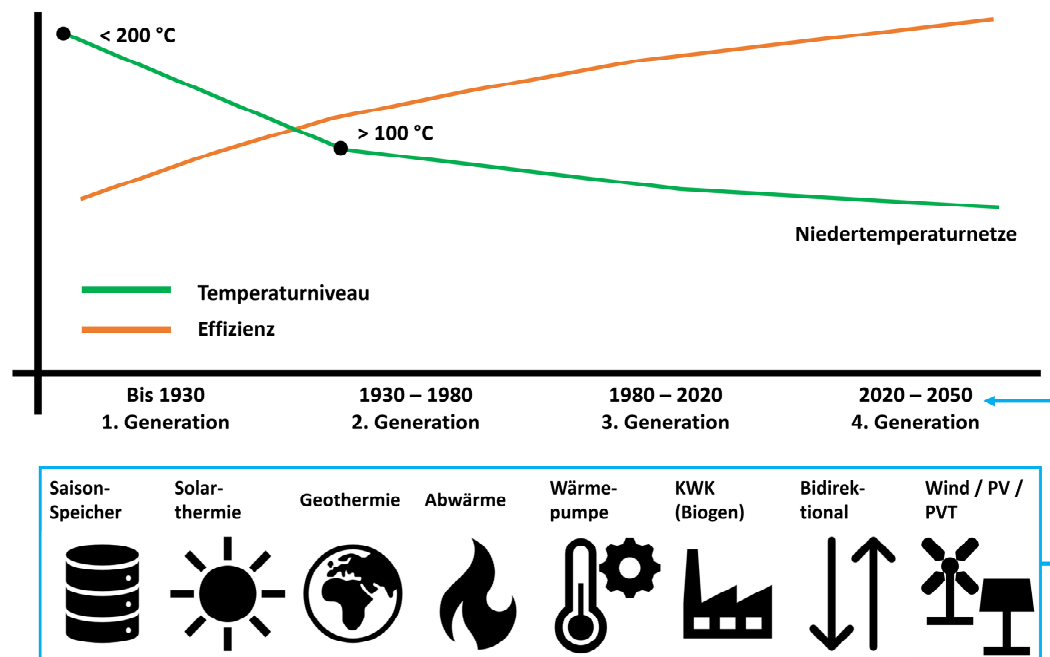
Abbildung 8: Wärmenetzgeneration und Entwicklung des Temperaturniveaus von der ersten bis zur vierten Generation nach Pehnt [14]
