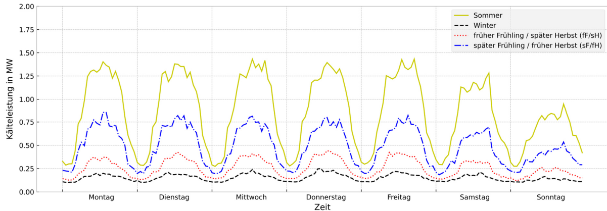
Abbildung 21: Typischer Wochen-Lastgang des Bürokomplexes für Kälte nach Bittner [62]
