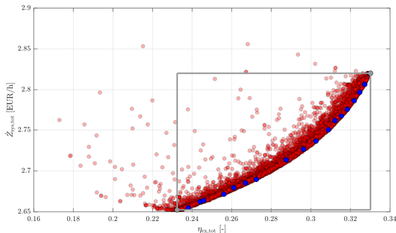
Abbildung 39: Pareto-Front der ersten Absorberschaltungsvariante für die reine Kältebereitstellung
