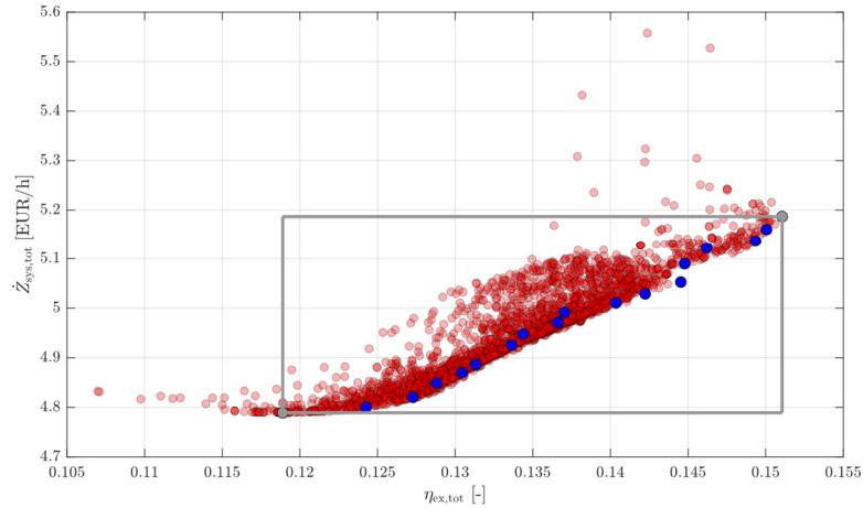
Abbildung 45: Pareto-Front der ersten Ejektorschaltungsvariante für die reine Kältebereitstellung
