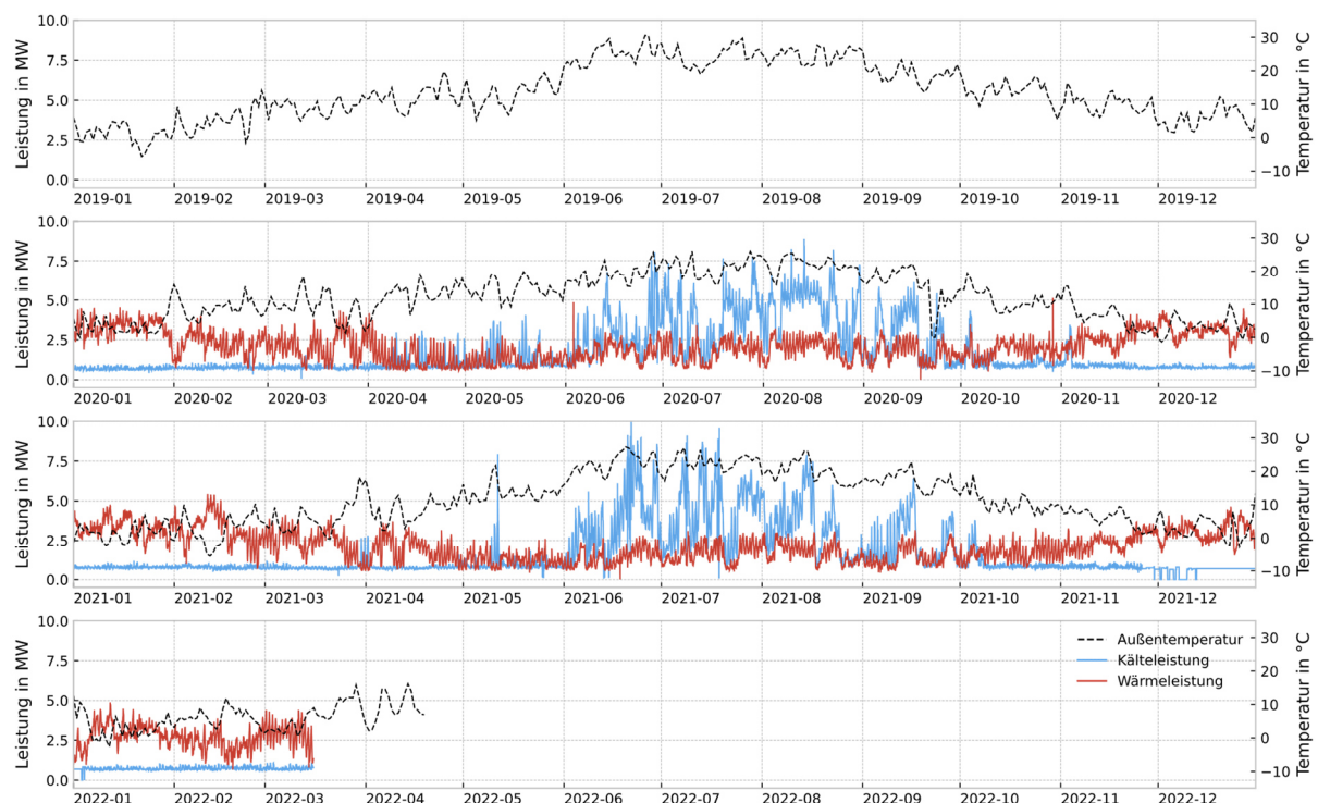
Abbildung 23: Lastgänge und Außentemperaturverläufe des Krankenhauses für 2019 bis 2022 nach Bittner [62]
