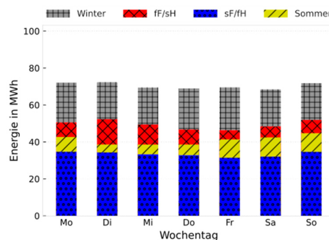
Abbildung 28: Typische tägliche Wärmeenergiemengen des Krankenhauses nach Bittner [62]
