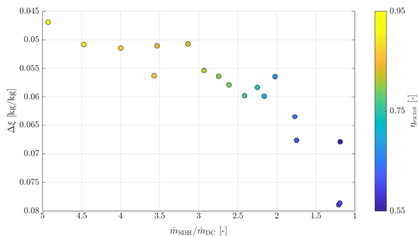
Abbildung 42: Parameterraum der zweiten Absorberschaltungsvariante für die simultane Wärme- und Kältebereitstellung
