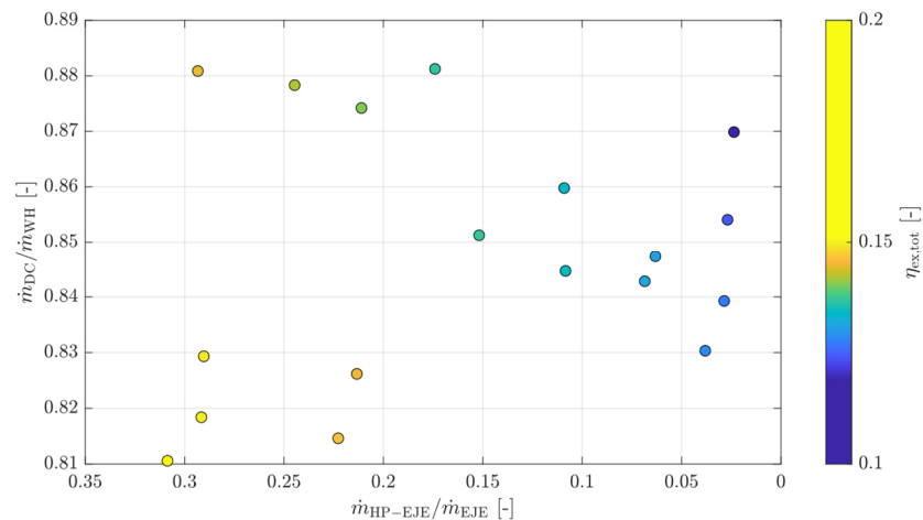
Abbildung 46: Parameterraum der ersten Ejektorschaltungsvariante für die reine Kältebereitstellung
