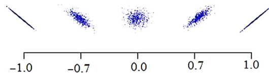
Abbildung 13: Veranschaulichung der Korrelation zweier numerischen Variablen nach Nettleton [66]
