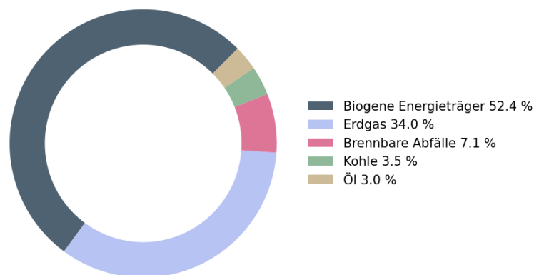
Abbildung 6: Anteile der Energieträger für die Nah- und Fernwärmeerzeugung in Österreich im Jahr 2020 nach dem Fachverband der Gas- und Wärmeversorgungsunternehmen [11]
