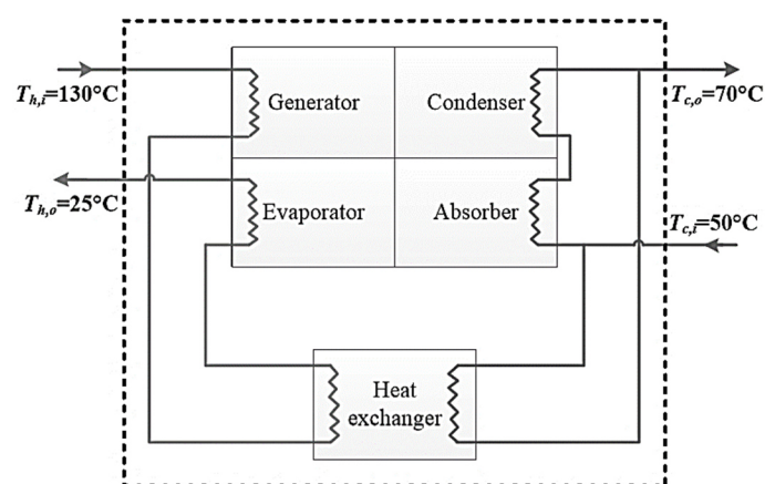
Abbildung 9: Schema eines Absorptionswärmetauschers nach Wu et al. [39]
