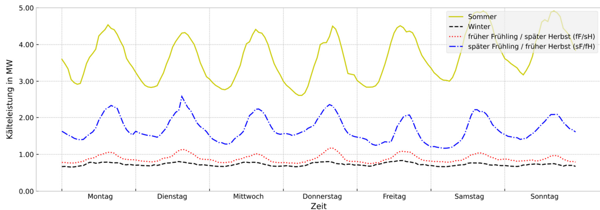
Abbildung 29: Typischer Wochen-Lastgang des Krankenhauses für Kälte nach Bittner [62]
