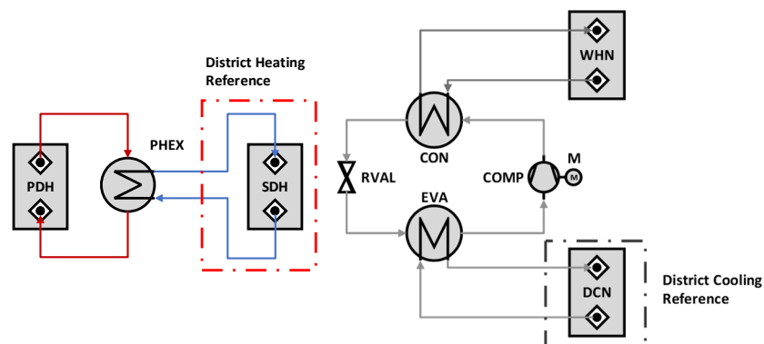
Abbildung 53: Schema des Referenzsystems im Falle der reinen Wärmebereitstellung
